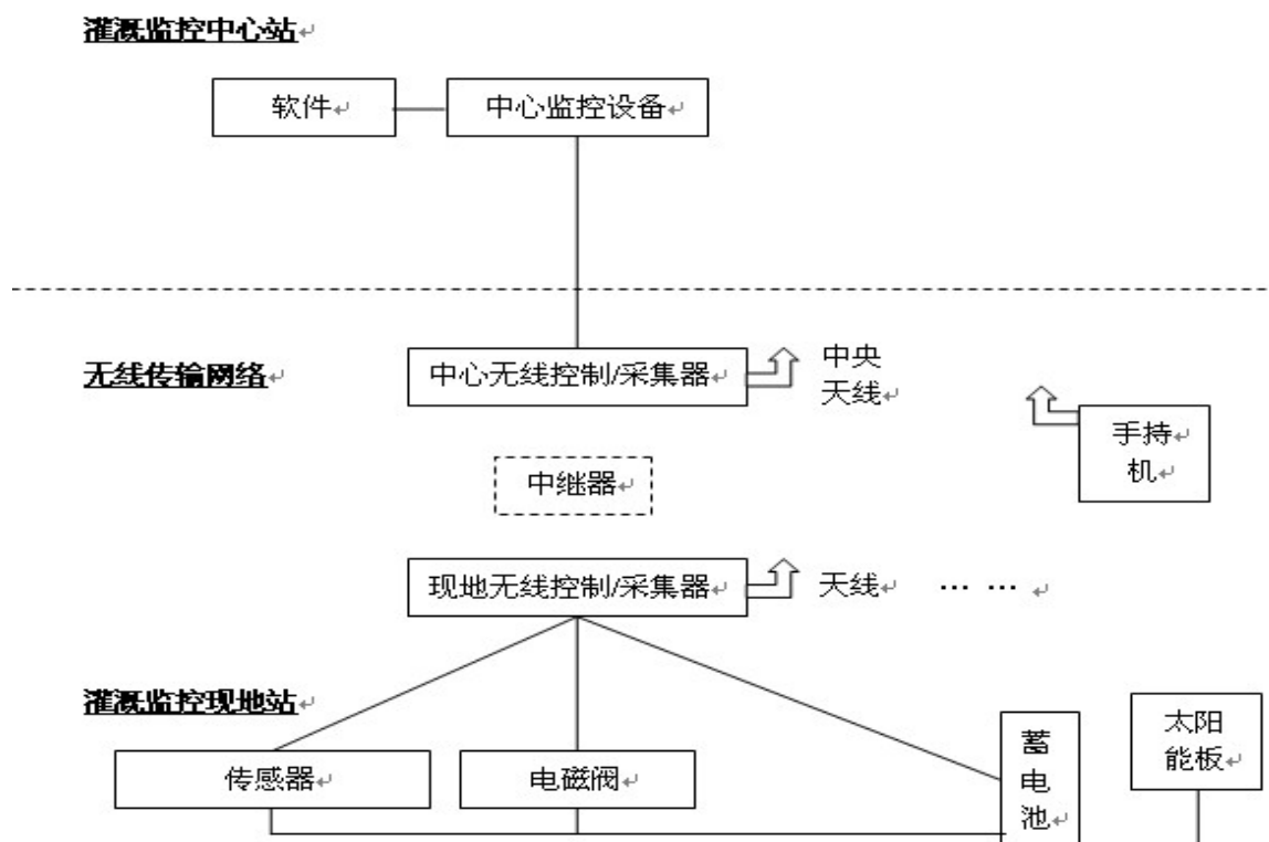
图2 节水灌溉太阳能无线智能控制系统基本结构组成示意图
