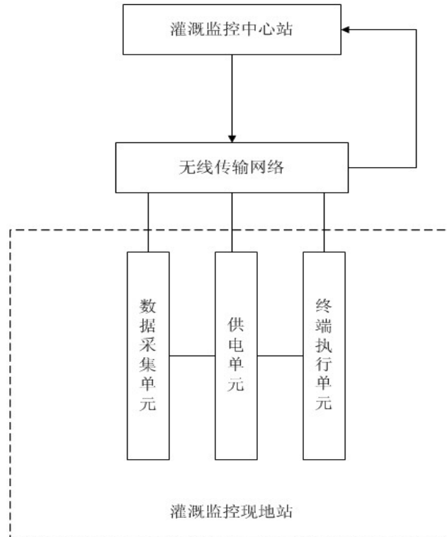
图1 节水灌溉太阳能无线智能控制系统单元组成示意图
